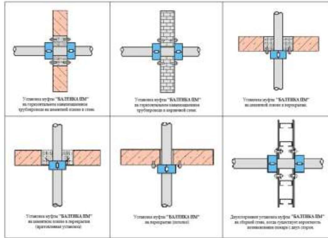
Схема установки 1
